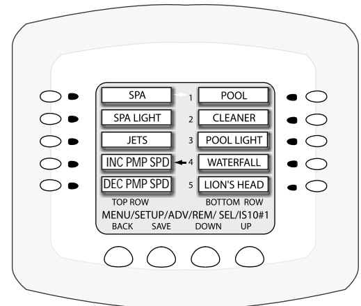
iS10 circuit/button setup
