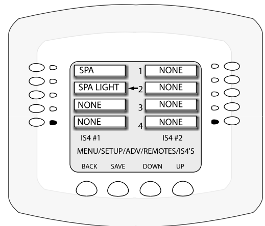
iS4 circuit/button setup
